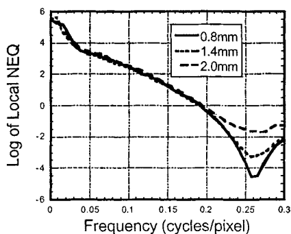
Fig. 13. The log values for the NEQ_r 's plotted in Fig. 12.
